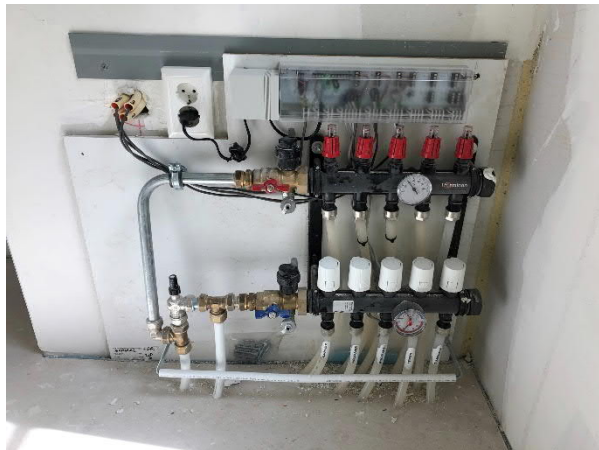
Vloerverdeling met ontluchting
