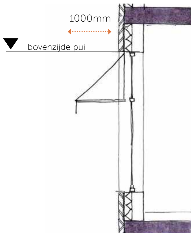
zijaanzicht valschermer
