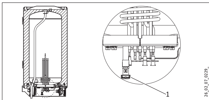
1 Capuchon de la vanne de vidange
